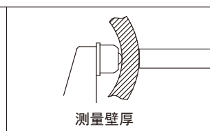
球测头(标配)
