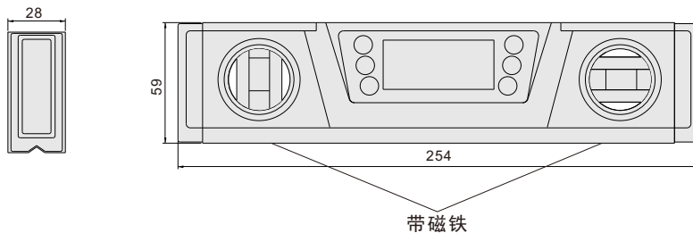
水平仪
