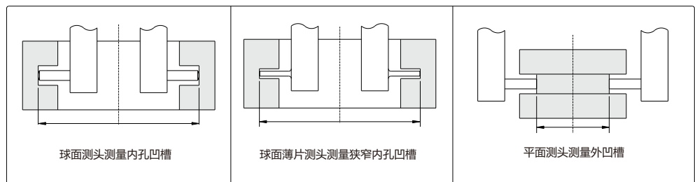
测量内凹槽和外凹槽
