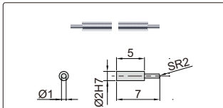
圆柱球面测头(标配)
