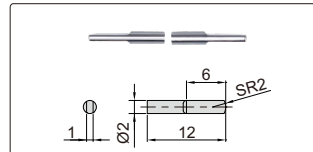
球面薄片短测头(标配)
