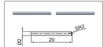
球面/平面长测头(标配)
