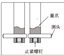
测头安装方式
