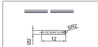
球面/平面短测头(标配)
