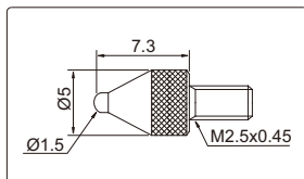
球形测针
